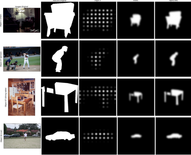
Figura 3: Ejemplo de percepciones simuladas para una misma máscara usando distintos modelos de implante. Las imágenes se renderizan en una grilla de 256 \times 256 píxeles para visualización, pero la información perceptual está limitada por la geometría del implante. En particular, Argus II posee 60 electrodos dispuestos aproximadamente en una grilla de 10 \times 6 , lo que ilustra la fuerte reducción de resolución respecto de la máscara original.
